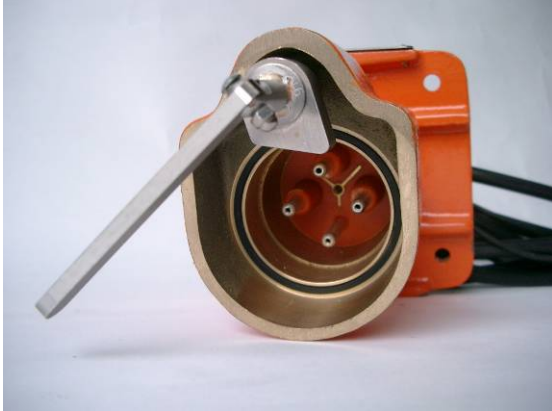
60 amp 660V Receptacle
